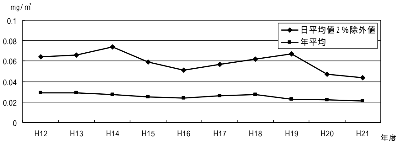
図3 - 4 浮遊粒子状物質(経年推移)
