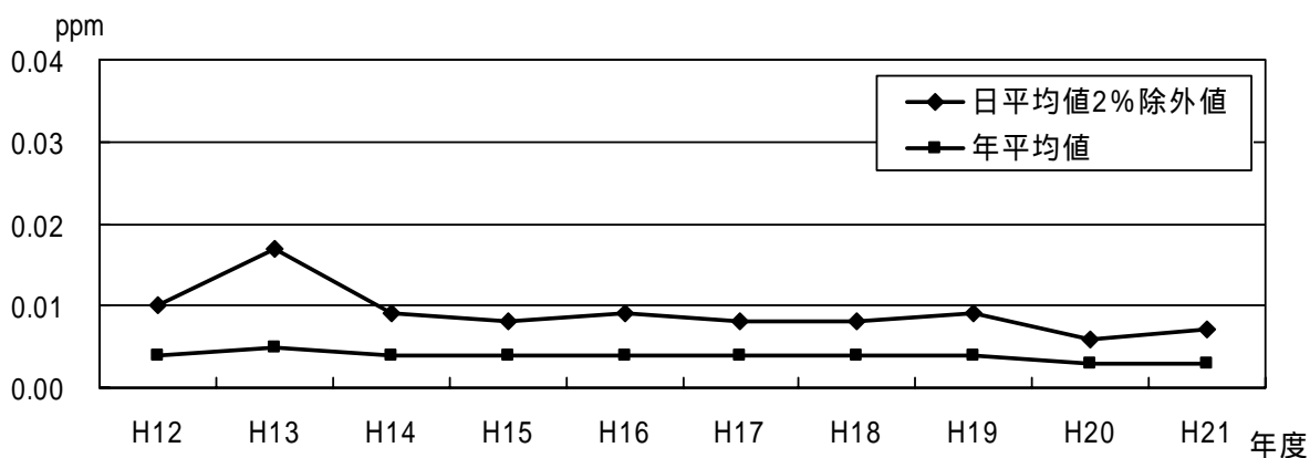
図3 - 5 二酸化硫黄(経年推移)
