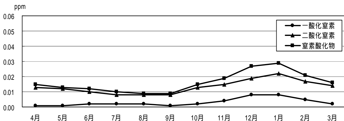
図3 - 1 窒素酸化物濃度の月平均値
