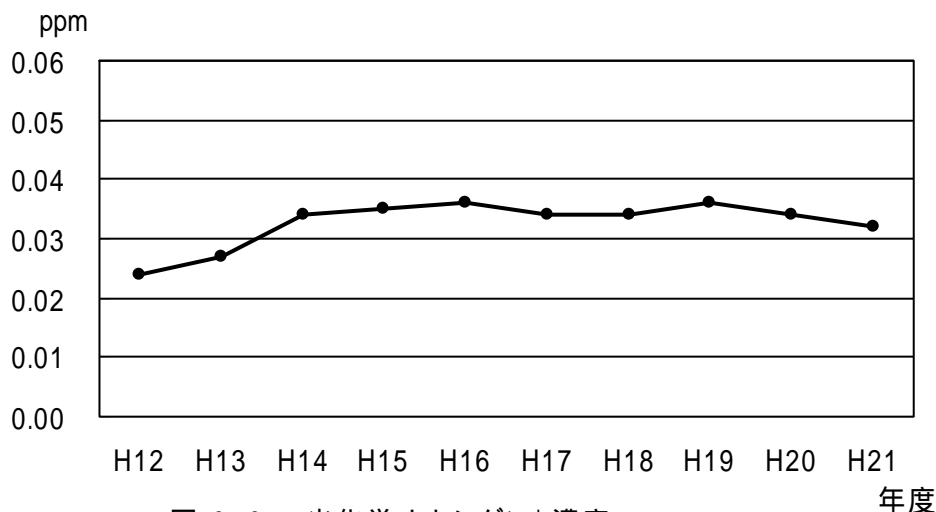
図3-3 光化学オキシダント濃度 昼間の1時間値の年平均値 (経年推移)
