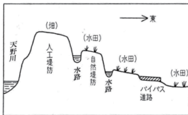
二重川断面模式図
