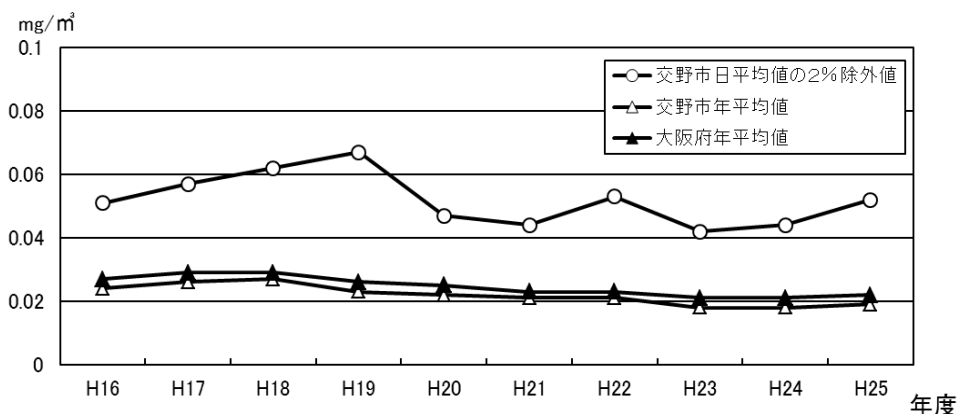
図3-4 浮遊粒子状物質濃度(経年推移)
