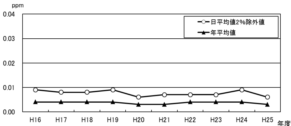
図3-5 二酸化硫黄濃度(経年推移)
