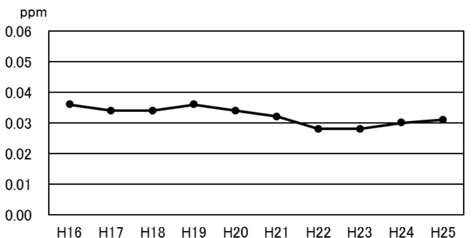
図3-3 光化学オキシダント濃度昼間年平均値(経年推移) 年度
