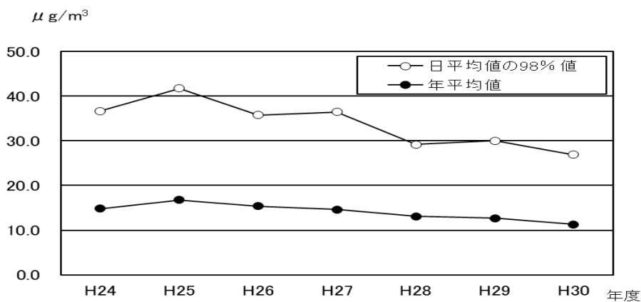
図3-5 微小粒子状物質濃度(経年推移・天野が原局)
