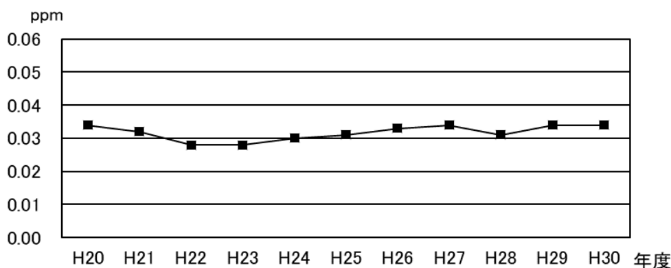
図3-3 光化学オキシダント濃度昼間年平均値 (経年推移・中央局)
