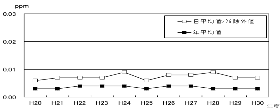
図3-6 二酸化硫黄濃度(経年推移・中央局)
