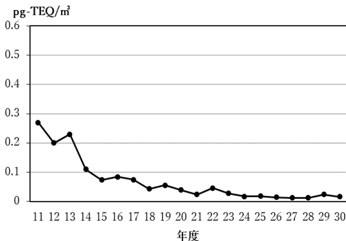
図 5-1 大気中ダイオキシン類(経年推移)
