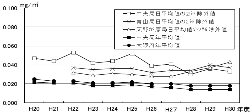
図3-4 浮遊粒子状物質濃度(経年推移)
