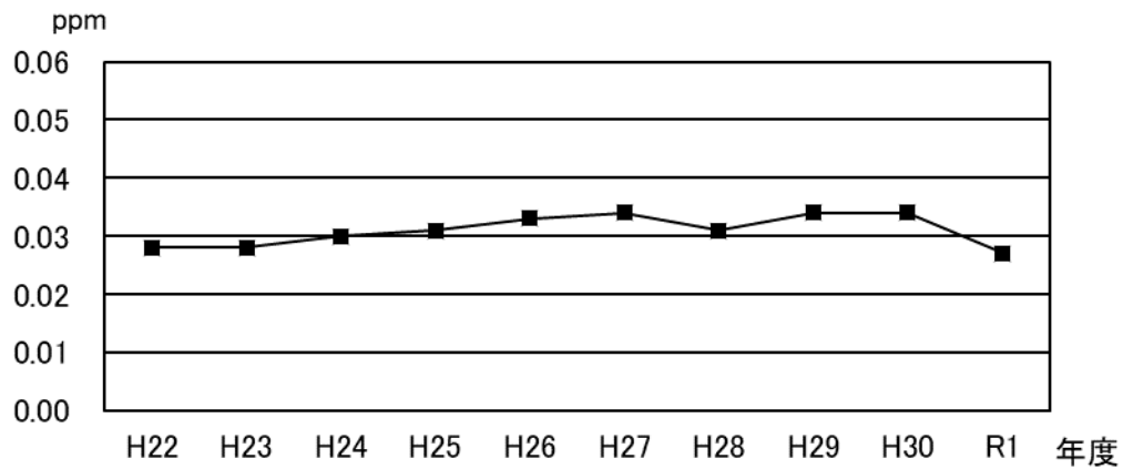
図3-3 光化学オキシダント濃度昼間年平均値（経年推移・中央局）
