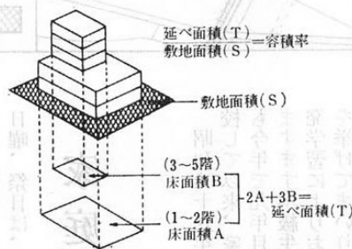
○建築物の容積率の例
