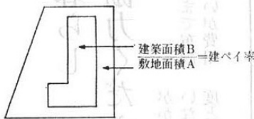
○建ぺい率による許容建築面積の例
