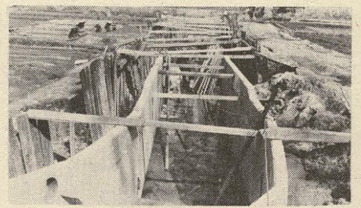
どろん川改修工事
