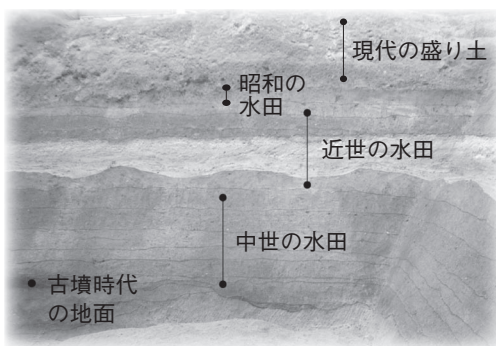
私部南遺跡の地層断面写真
