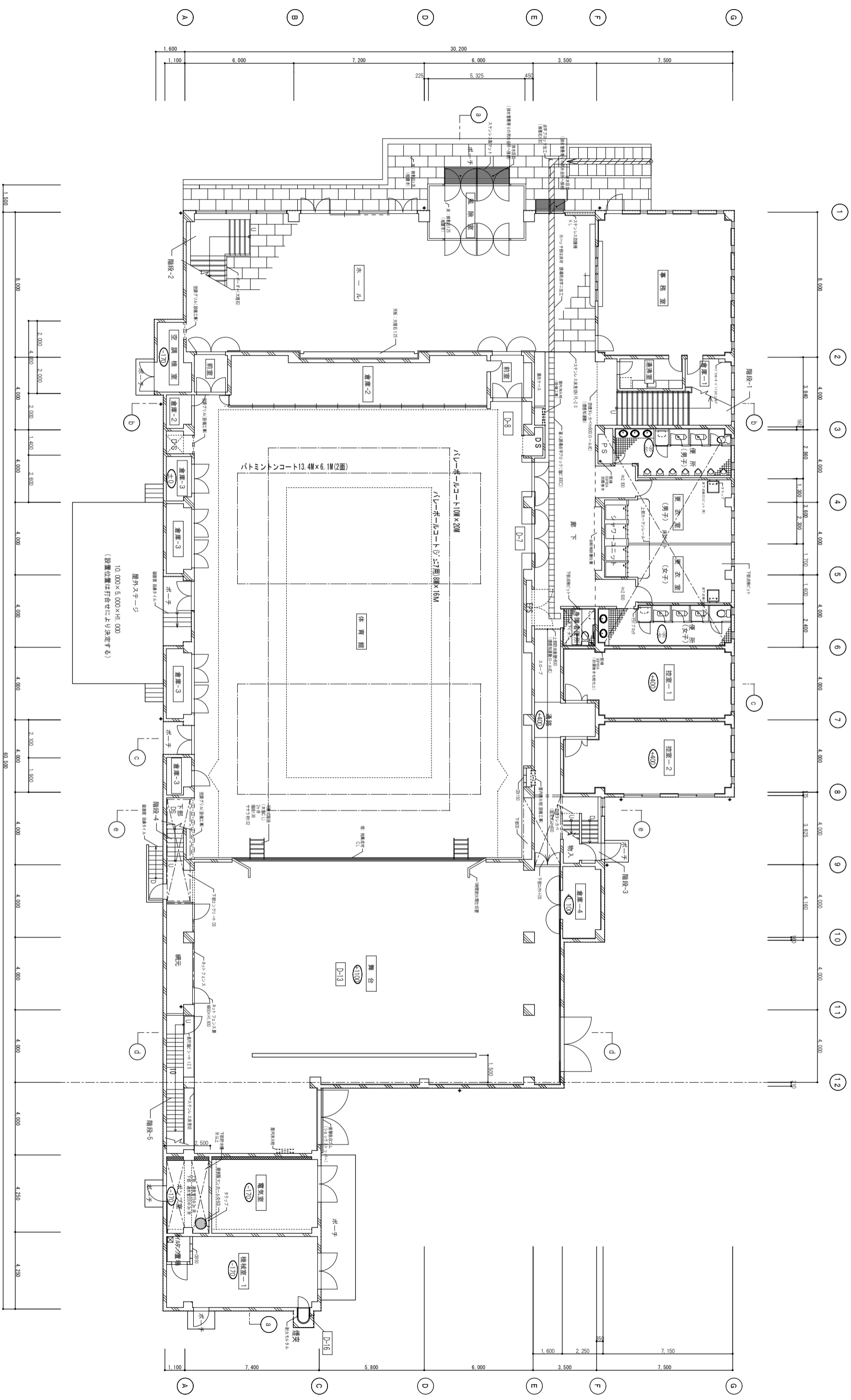
1 階 平 面 図 1/200
