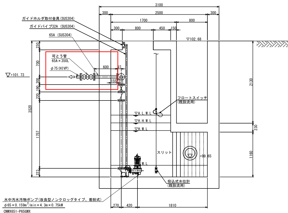
A - A 断面図 S=1:25
