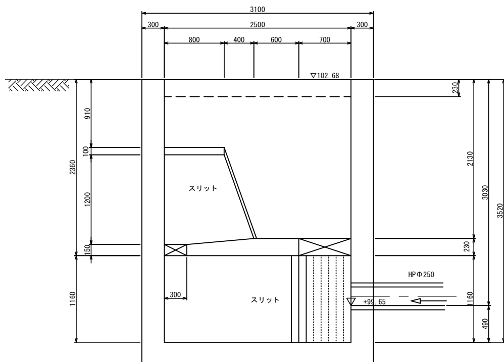
B - B 断面図 S=1:25
