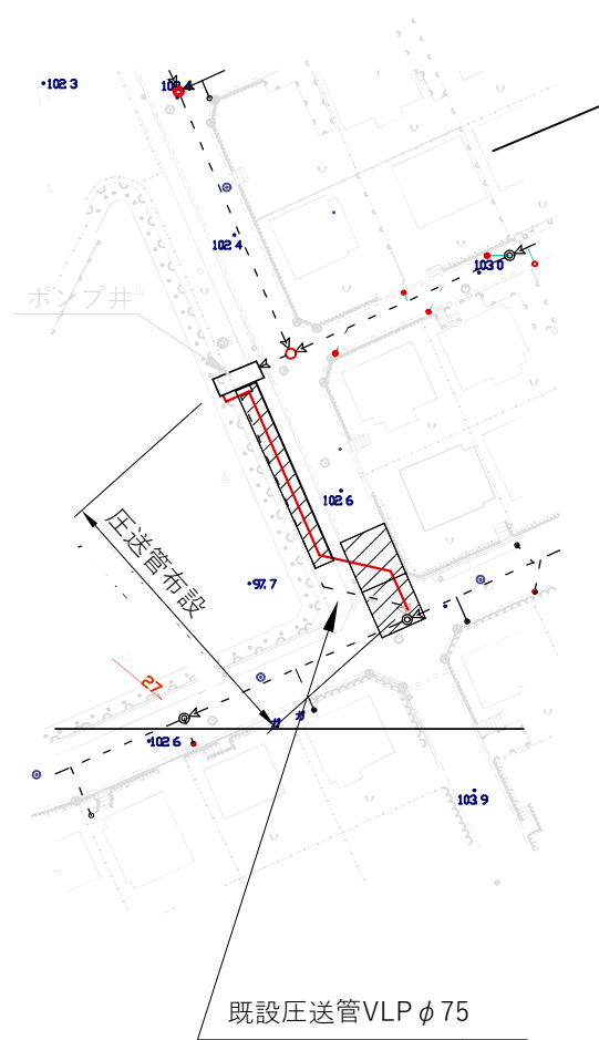
平面図
