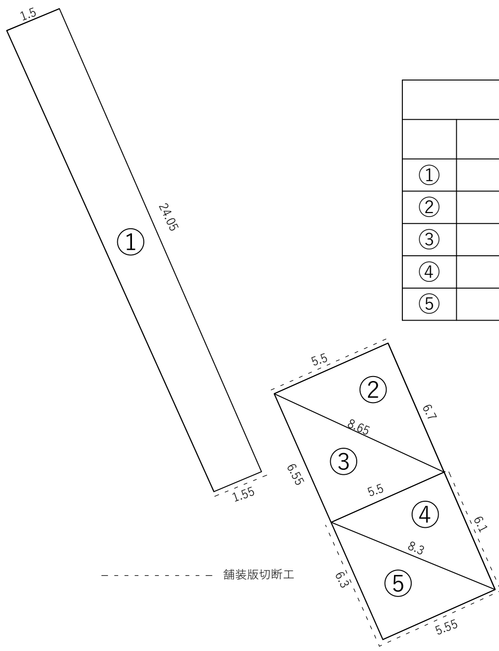
舗装復旧展開図
