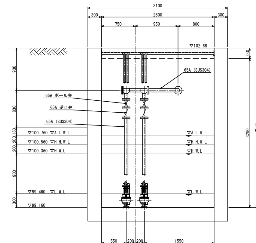
C - C 断面図 S=1:25
